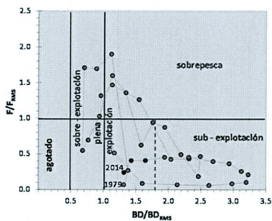
Figura 1. Diagrama de fase de langostino amarillo área sur. El PBR corresponde a un F = 45\%SPR . La biomasa objetivo equivale a un 45\%SPR ( 40\%Bo ). La razón B_{2014}/B_{RMS} = 1,32 y F_{2014}/F_{RMS} = 0,24 .
